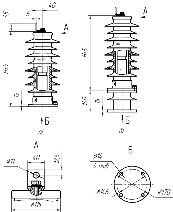
Рис. 2. Ограничитель перенапряжений нелинейный типа ОПН – У – 27 (35)
