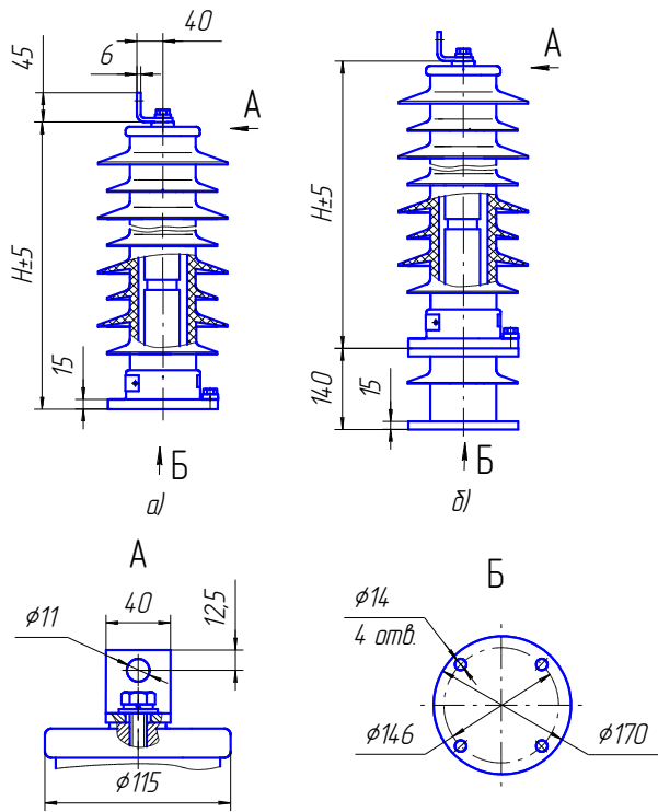
Рис. 2. Ограничитель перенапряжений нелинейный типа ОПН – У – 15 (20)
