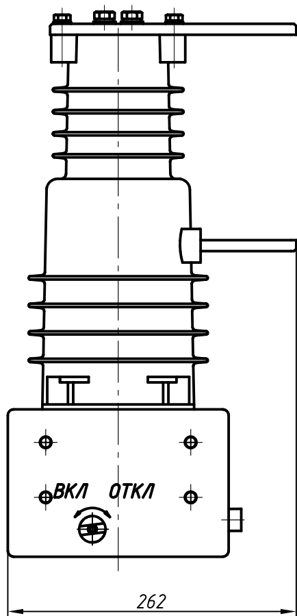
Вакуумный выключатель BB/AST-10-20/1000-UHL2 исп.01
