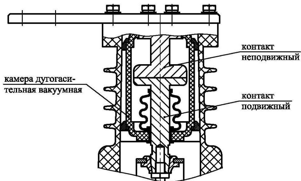
ВЫКЛЮЧАТЕЛЬ ВКЛЮЧЕН
