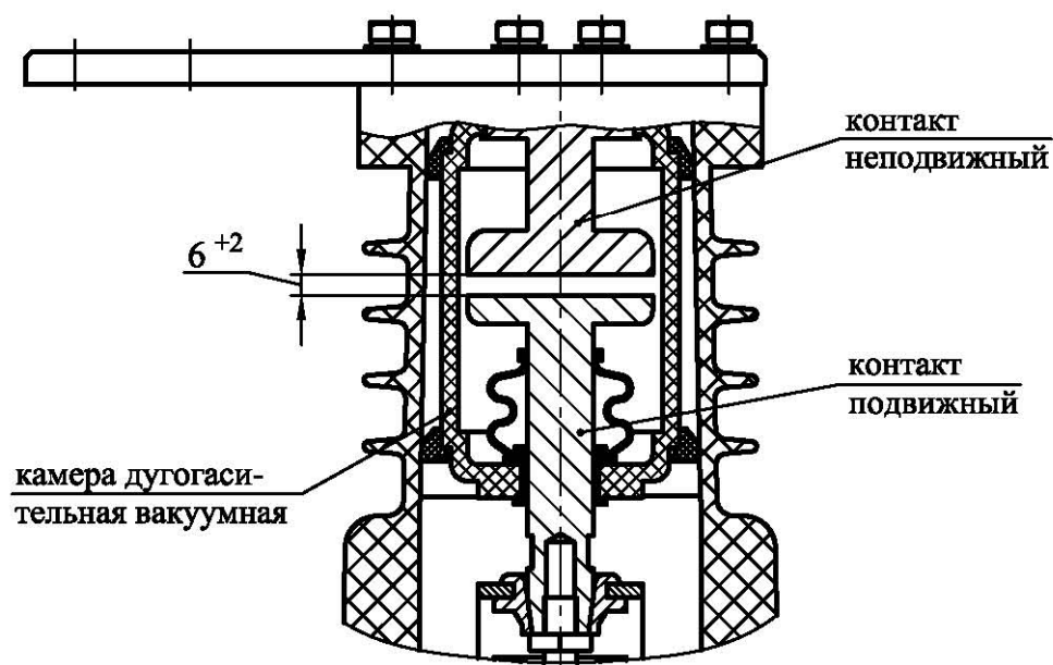
ВЫКЛЮЧАТЕЛЬ ВЫКЛЮЧЕН
