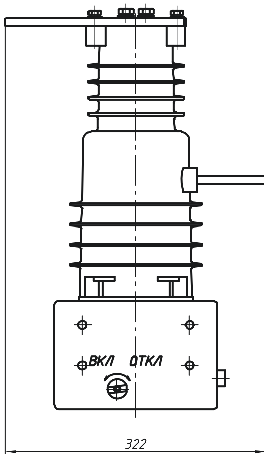
Вакуумный выключатель BB/AST-10-20/1000-UHL2 исп.03
