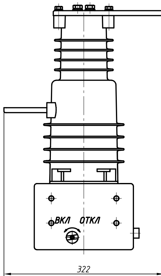
Вакуумный выключатель BB/AST-10-20/1000-UHL2 исп.02
