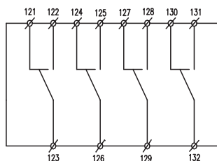
Электрическая схема
