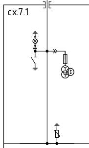
Шкаф с измерительным тр-ом Ввод/вывод ВЛ
