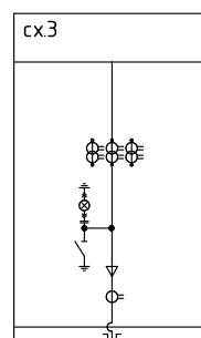
Шкаф Ввода/вывода кабелем снизу
