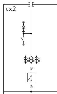
Шкаф с силовым выключателем Ввод/вывод ВЛ
