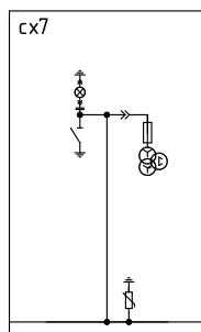
Шкаф с шинным заземлителем и измерительным тр-ом
