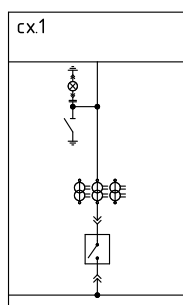
Шкаф с силовым выключателем и трансформаторами тока Ввод/вывод шинами сверху
