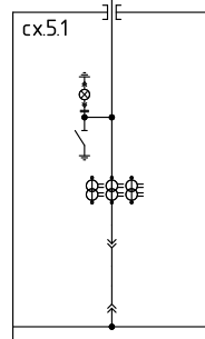
Шкаф с разъединителем Ввод/вывод ВЛ
