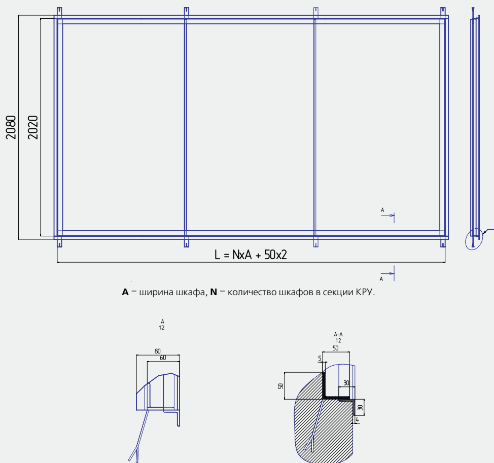
Рис. 16 Пример конструкции фундаментной рамы
