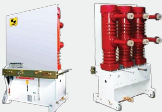
Рис. 8 Выдвижной элемент с выключателем VD 4.
